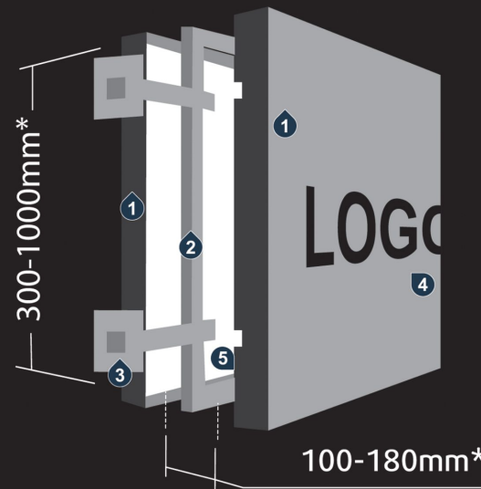
Profil DS (Dobbelsidig)
